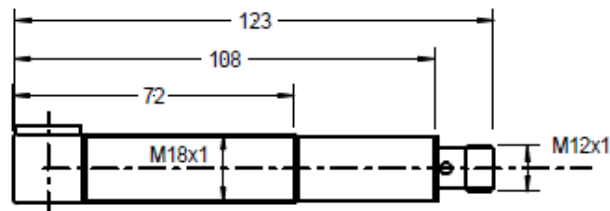
UFA-1500-M18-AR / UFA-1500-M18-1PR: radiale Messrichtung
