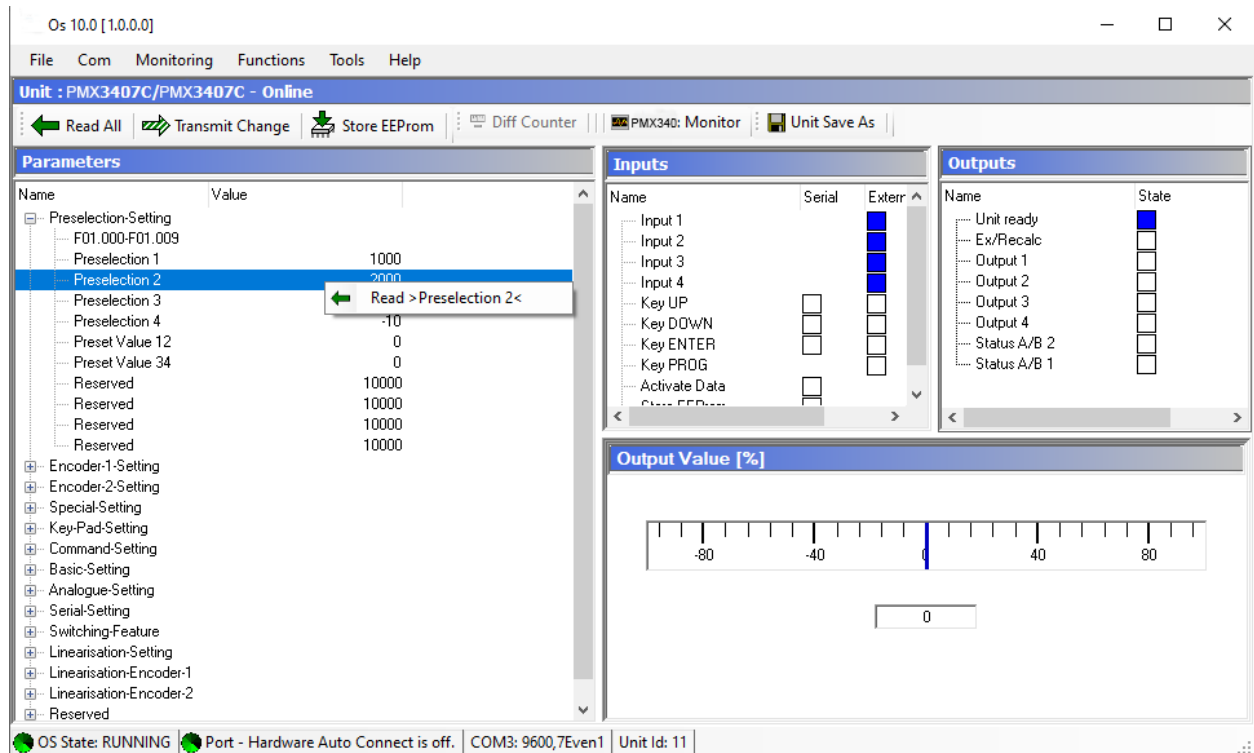
Abbildung 2-3 Parameter-Liste - PMX340
