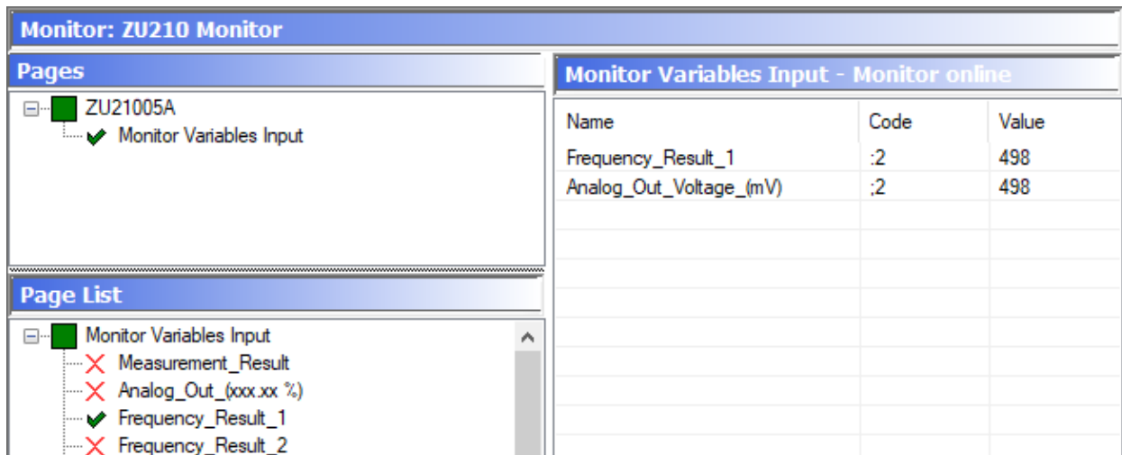
Abbildung 2-32 Monitor / Monitor Online - Beispiel
