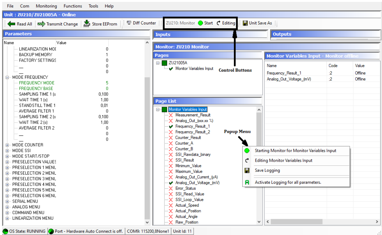
Abbildung 2-27 Monitor / Popup-Menü und Control-Buttons
