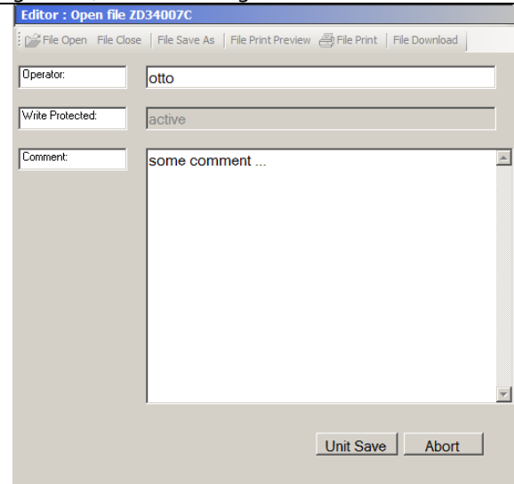
Abbildung 4-13 File Editor: Änderungsfenster (mit „Write Protected“)
