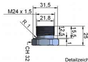
Detailzeichnung Gewindeflansch
