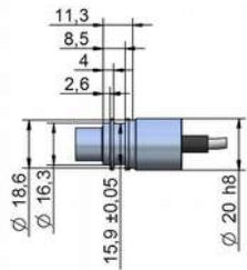
Detailzeichnung Steckflansch
