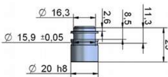
Detailzeichnung Steckflansch
