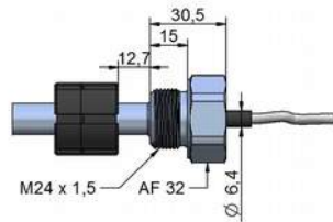
Detailzeichnung Steckflansch
