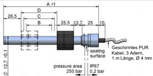
Detailzeichnung Gewindeflansch
